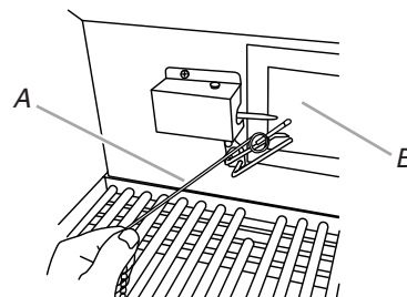
A. Porte-allumette
